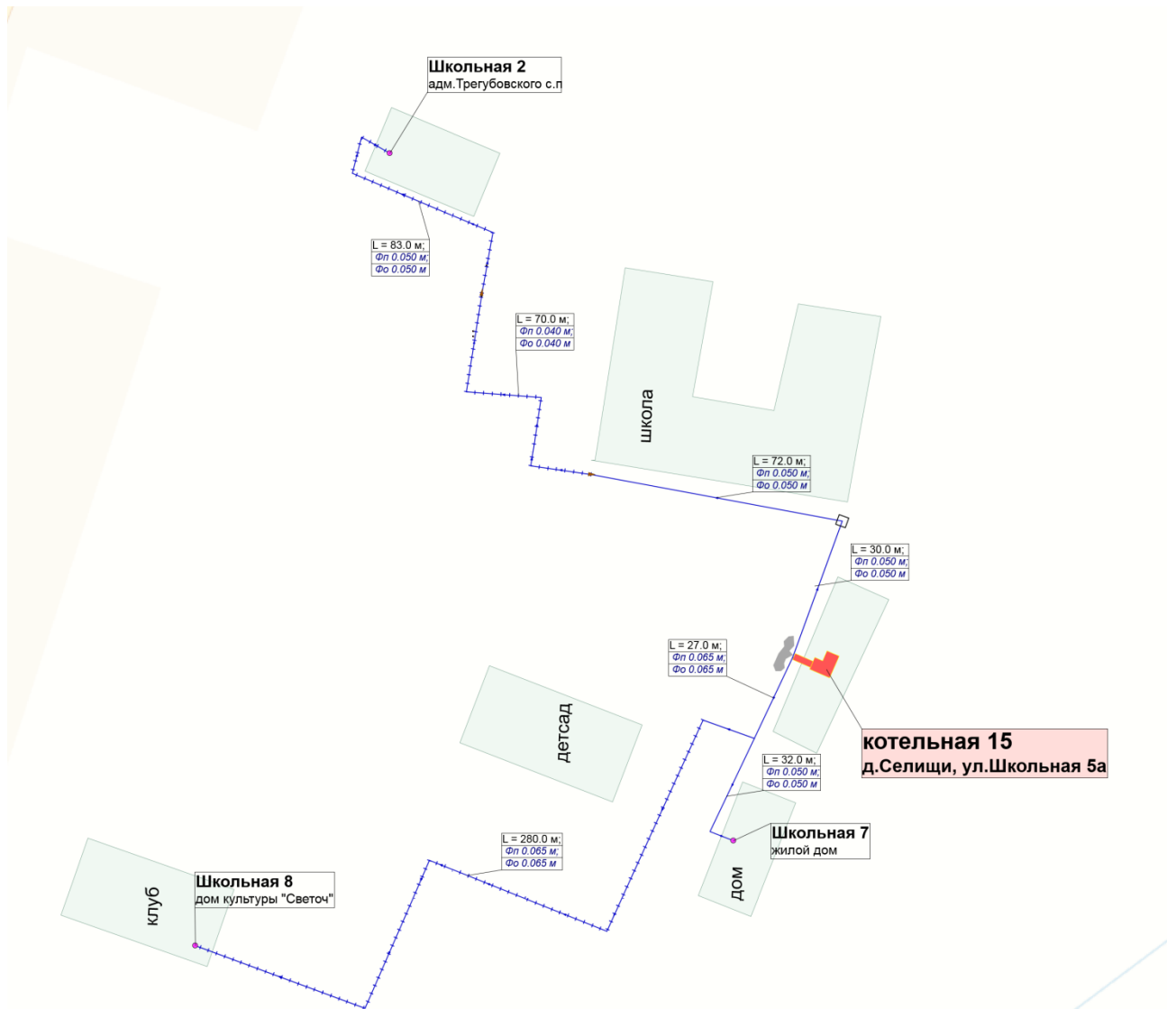
Рисунок 1.2. Схема тепловых сетей котельной № 15 д.Селищи
